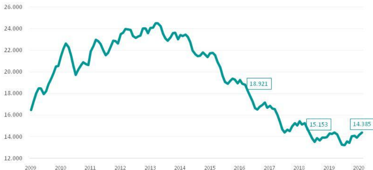
Gràfic 3. Evolució mensual del nombre d'ATURATS registrats a l'Hospitalet. 2009-2020. En nombre
