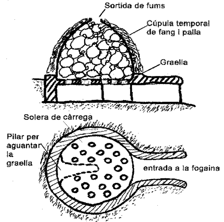
Fig. 2 Forn de terrissa antic
