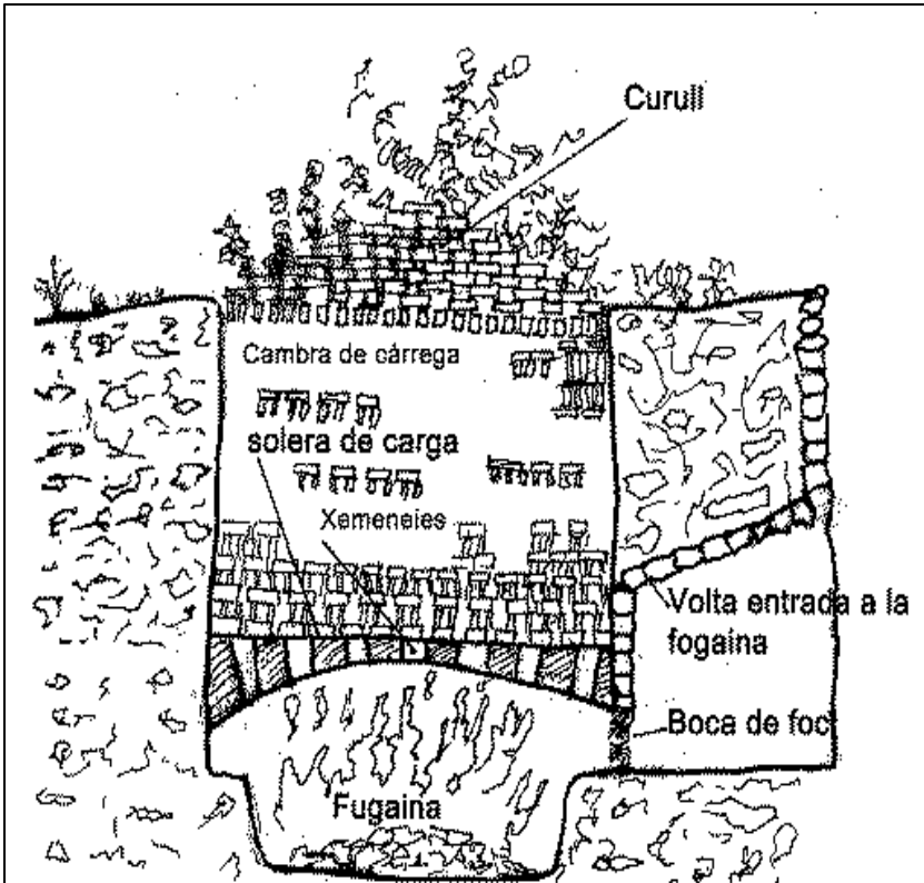
Fig. 3 Forn de rejoleria
