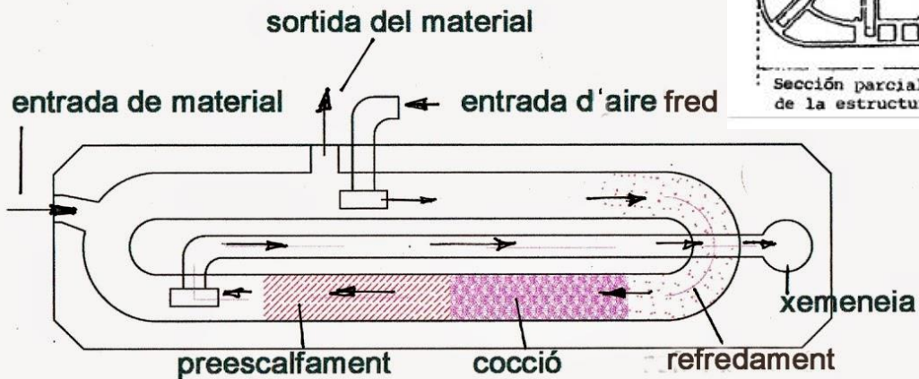
Fig.4 Forn de túnel
